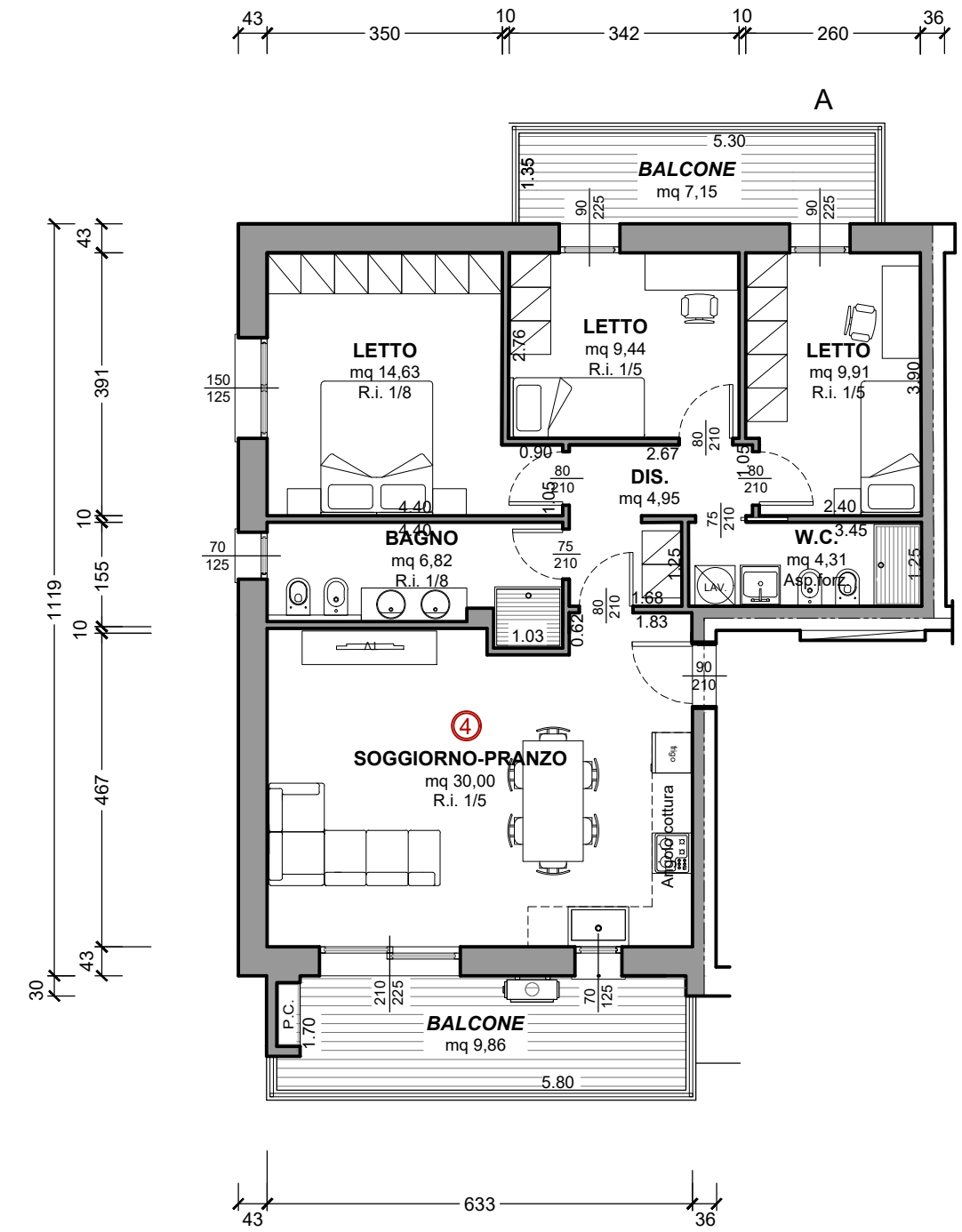
PIANTA PIANO PRIMO sc.1:100
