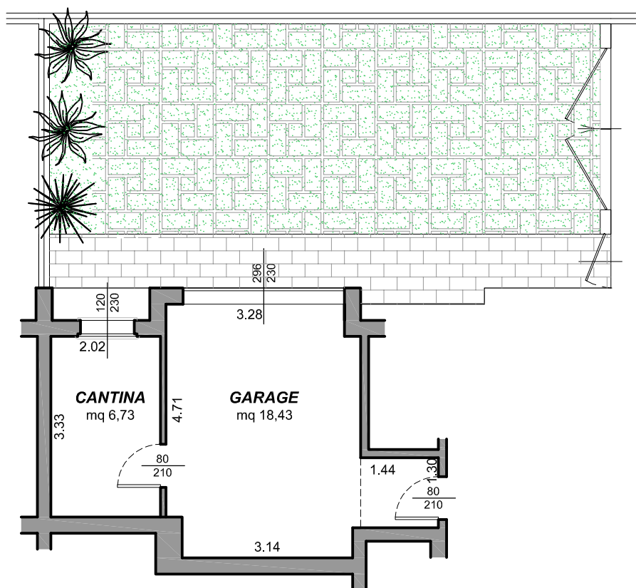
PIANTA PIANO TERRA sc.1:100
